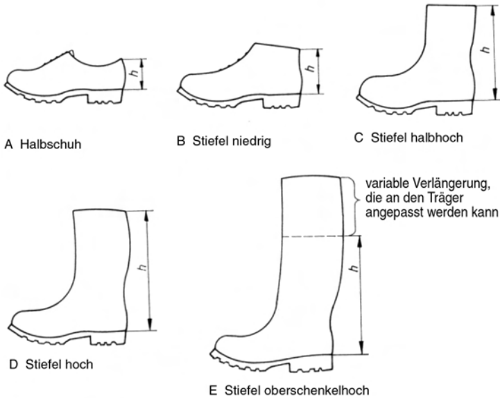
Bild 3: Schuhformen
