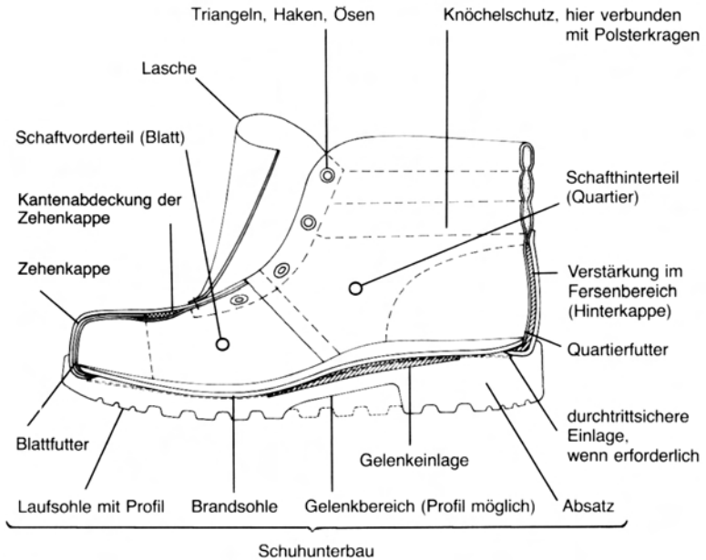
Bild 1: Beispiele für Bestandteile eines Schuhs
